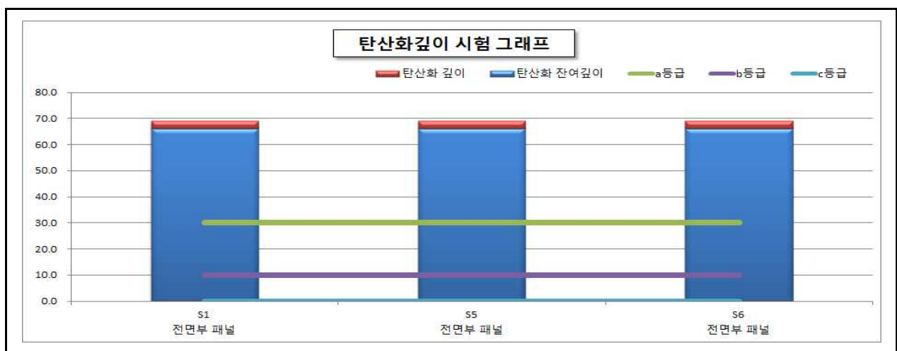
【그림 79.8】 탄산화 깊이 측정결과
